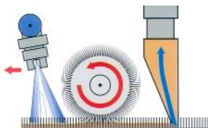
Sistema iniezione-estrazione con spazzola rotante
